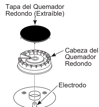
Quemador Redondo
