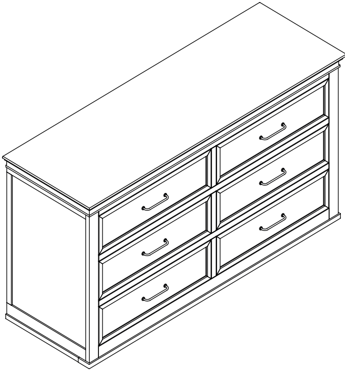
A-1. Dresser Body A-1. Cadre de la commode
