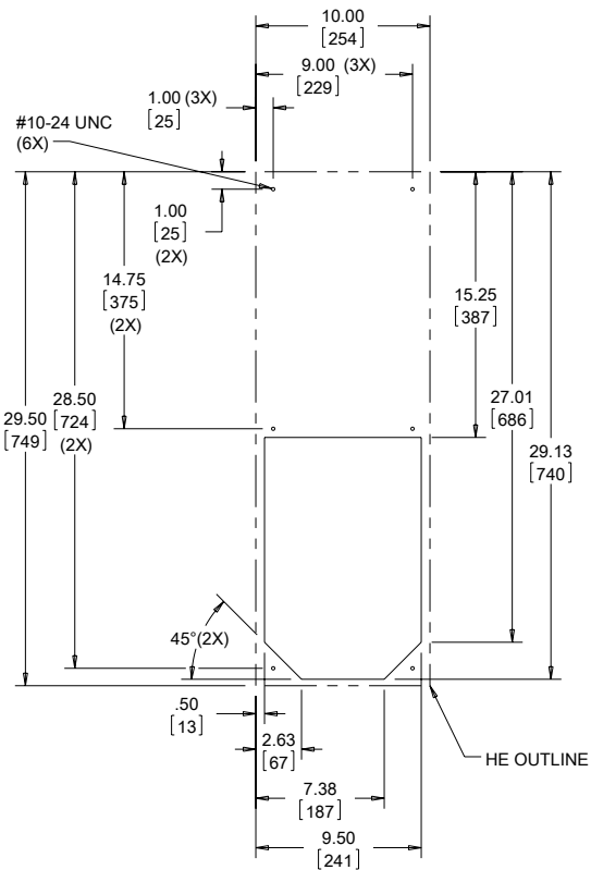
Cutout Dimensions
