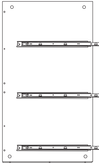
B-2. Right side B-2. Panneau latéral droit
