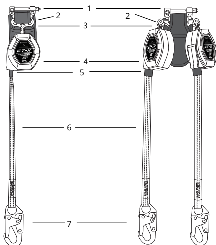
Figura 2 - Sobre la Cuerda de Salvamento Autorretráctil-P FT-X EdgeCore, Arco Eléctrico, Bordes Salientes Clase 2
