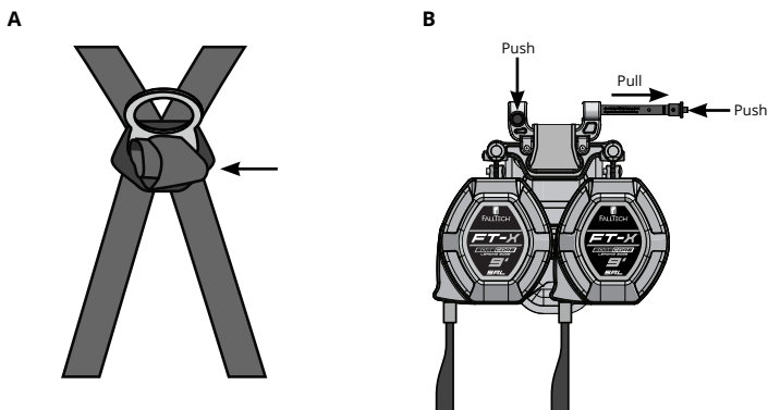
Figure 5 - Installation du bord d'attaque SRL-P de classe 2 FT-X EdgeCore à arc électrique
