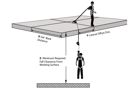
Figura 14 - Distancia despejada de caída mínima requerida de FT-X para usuarios de 310 a 420 libras (141 a 191 kg)
