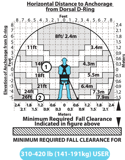
Figure 14 - Dégagement de chute minimum requis pour le FT-X pour les utilisateurs de 141 à 191 kg (310 à 420 lb)
