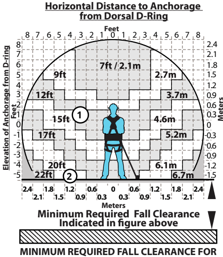
Figura 11 - Distancia despejada de caída mínima requerida de FT-X para usuarios de 130 a 310 libras (59 a 141 kg)
