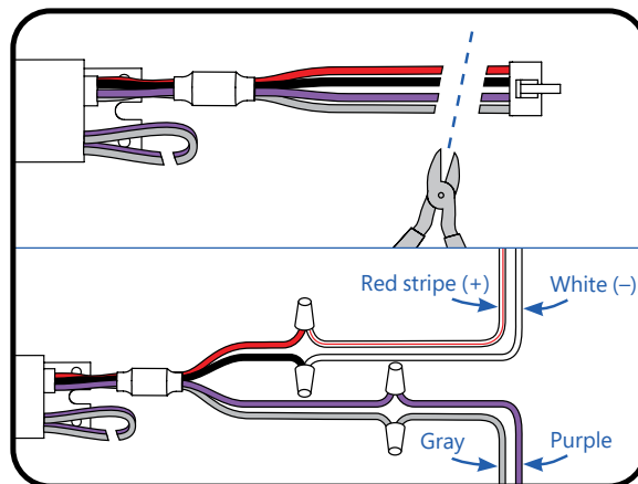
(D) Connect DC output using wire nuts.
