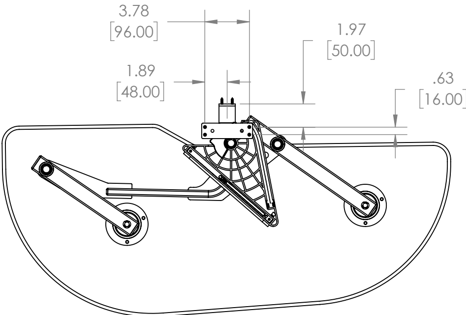
BOTTOM VIEW SCALE: 1/8
