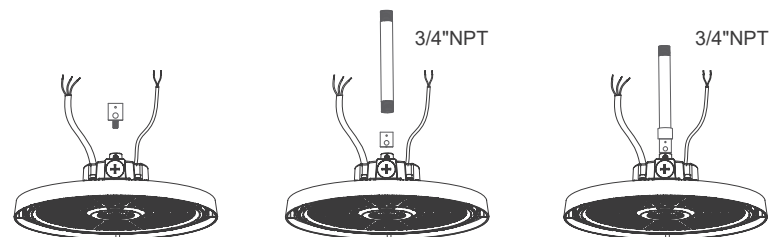
Pendant Mount
